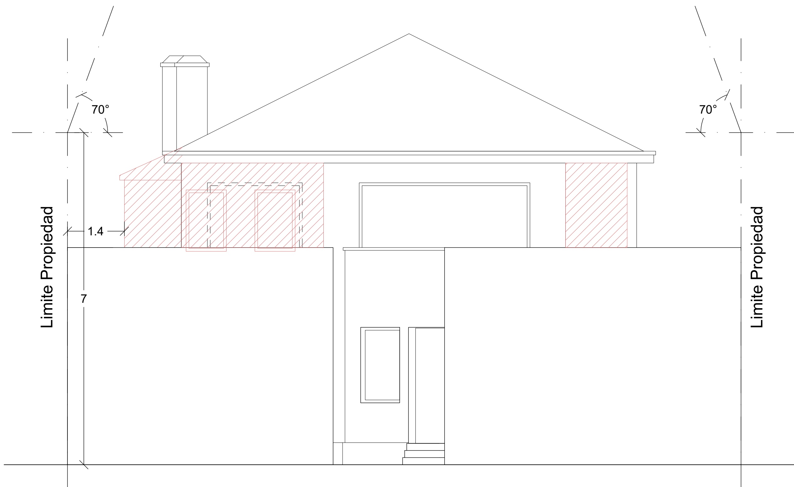
Elevación Sur Esc. 1:50
