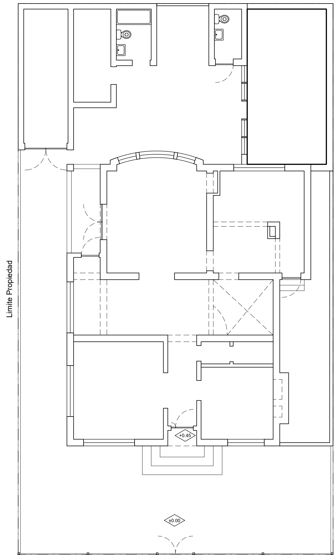
Situacion Existente Nivel 1 Esc. 1:100
