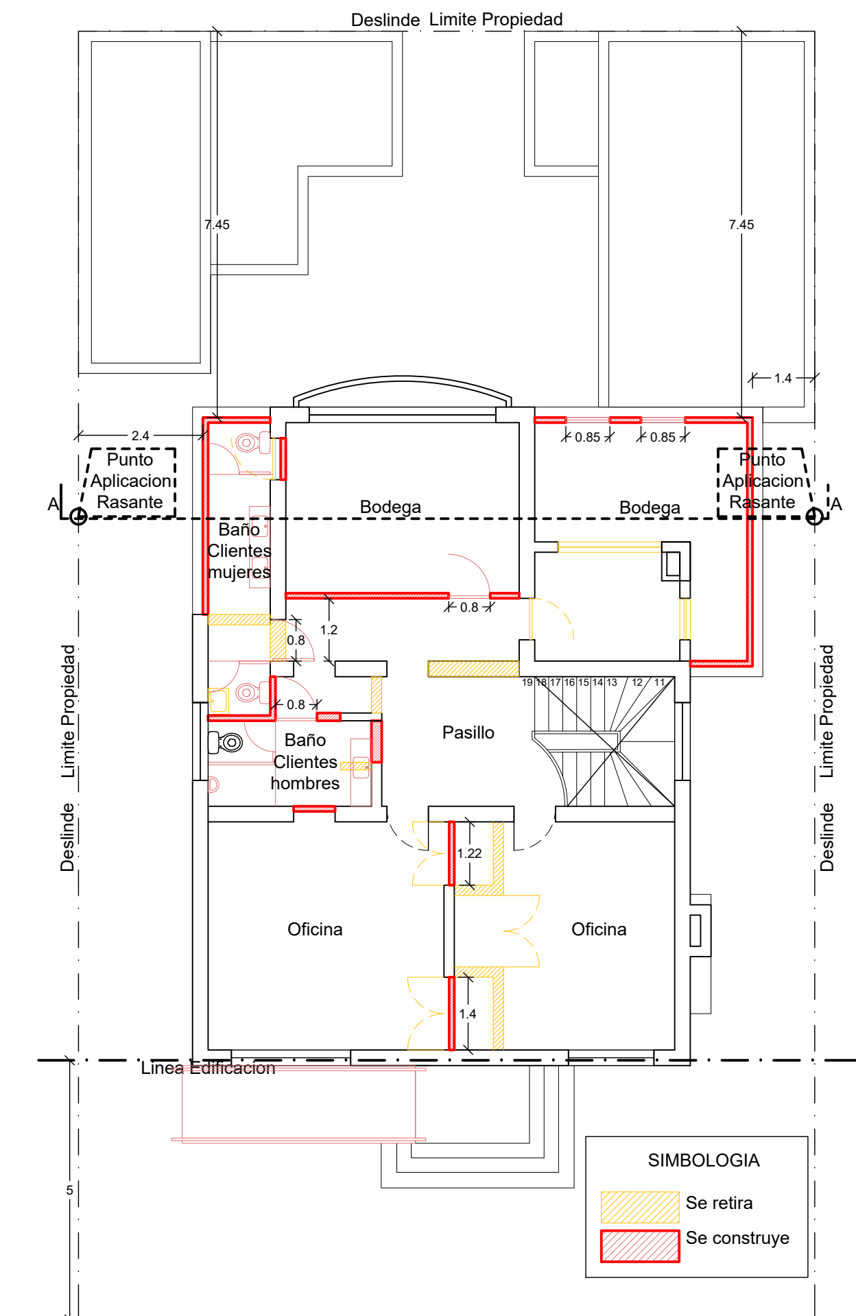
Situacion Propuesta Nivel 2 Esc. 1:100
