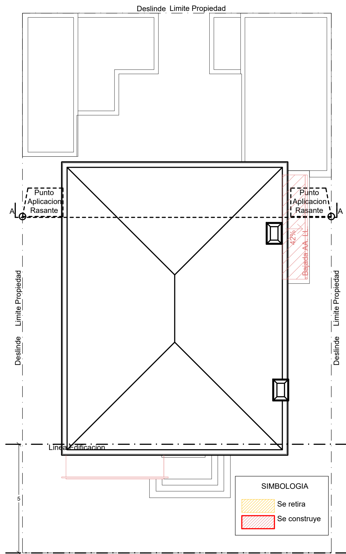
Situación Propuesta Cubiertas Esc. 1:100
