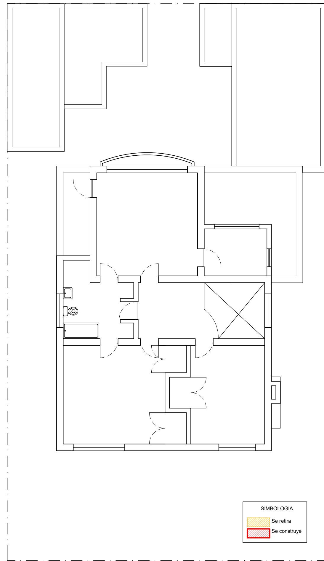
Situacion Existente Nivel 2 Esc. 1:100
