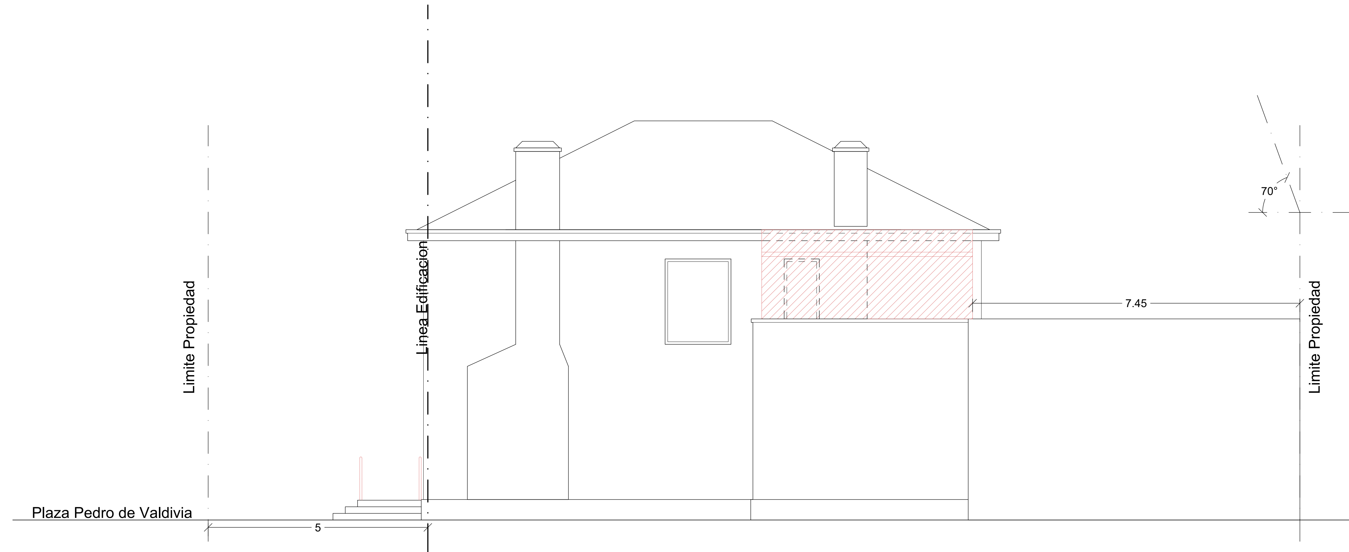
Elevación Oeste Esc. 1:50
