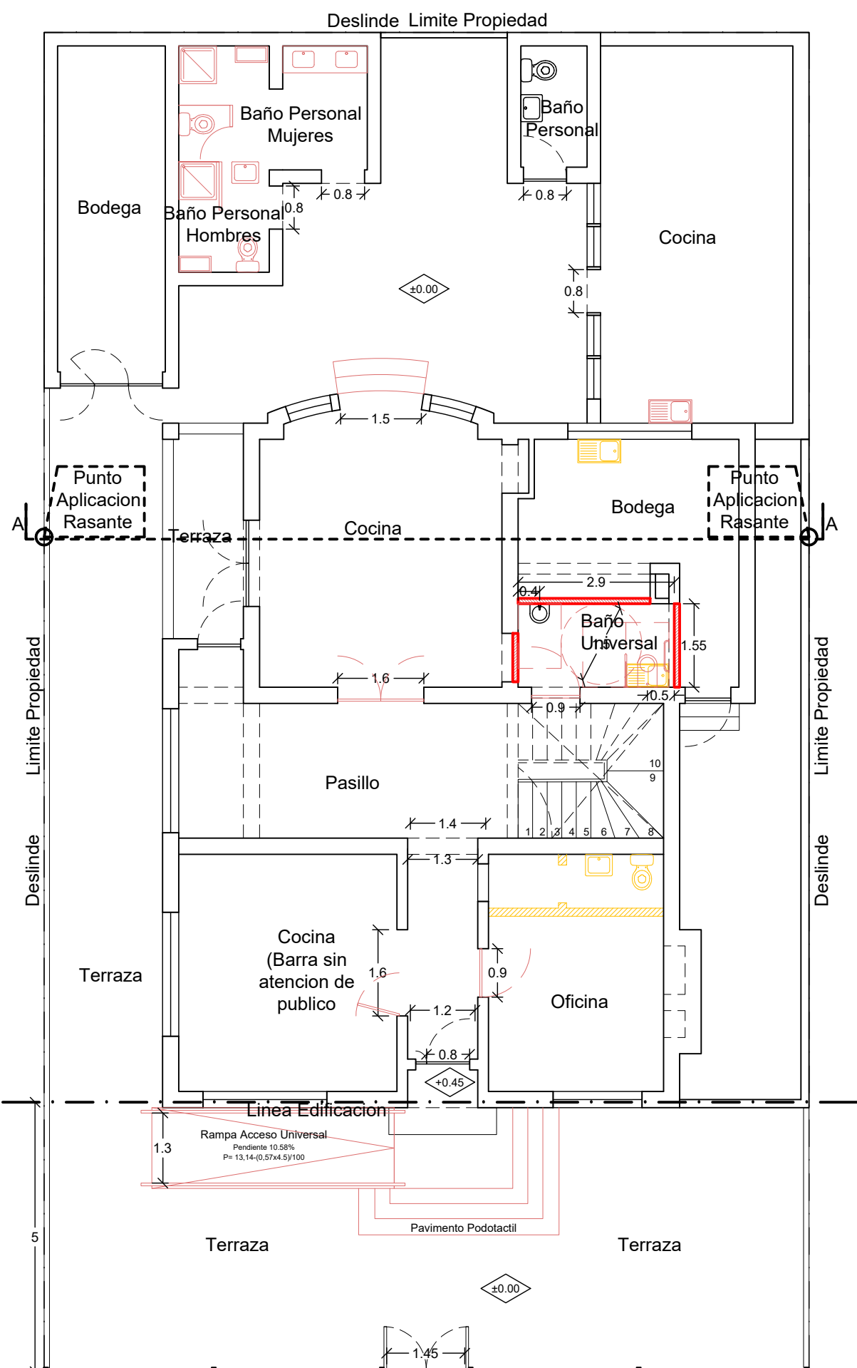
Situacion Propuesta Nivel 1 Esc. 1:100
