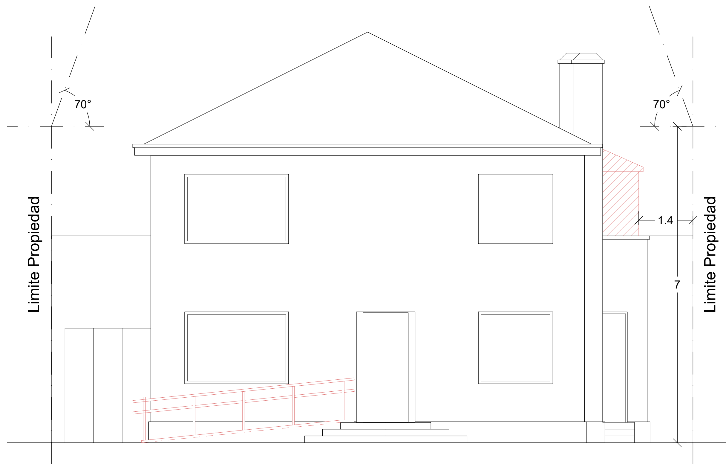
Elevación Norte Esc. 1:50
